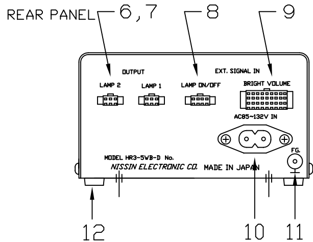
後面 REAR PANEL
