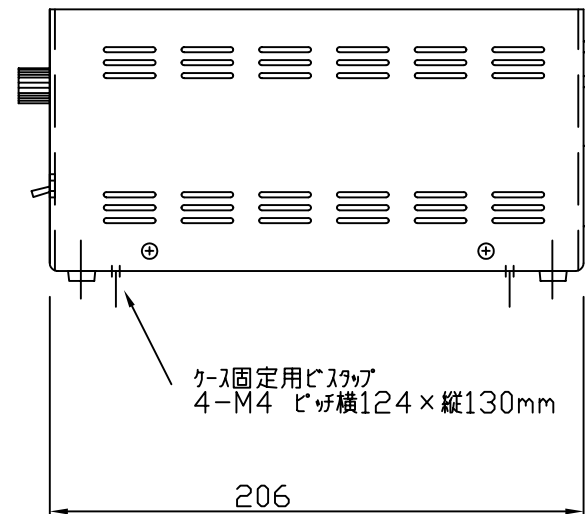
側面
