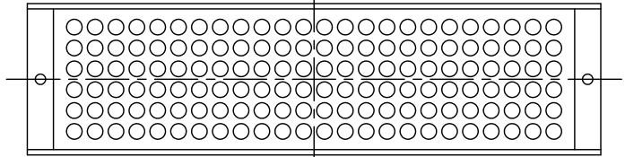
赤, 赤外 照明 24個x6列 (素子間P=4mm)
