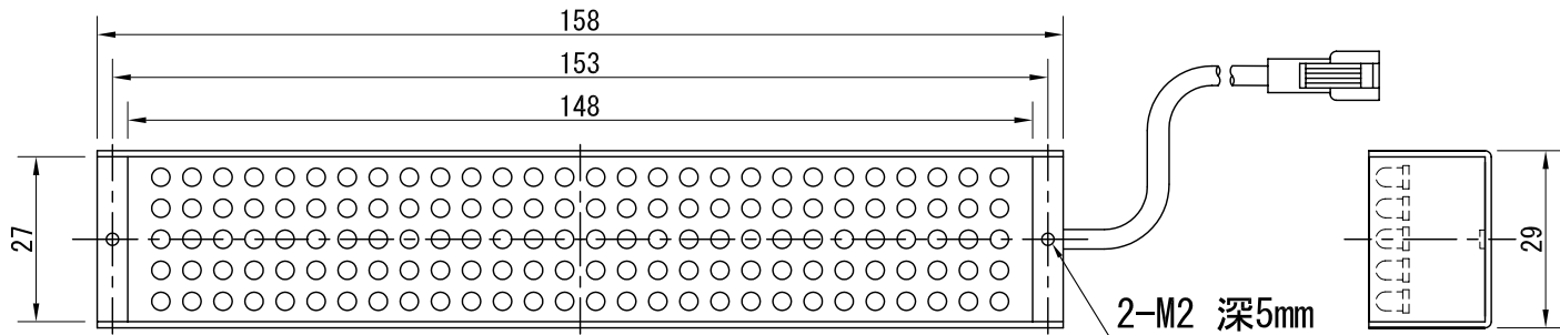
白, 青, 緑, 紫外 照明 28個x5列 (素子間P=5.08mm)
