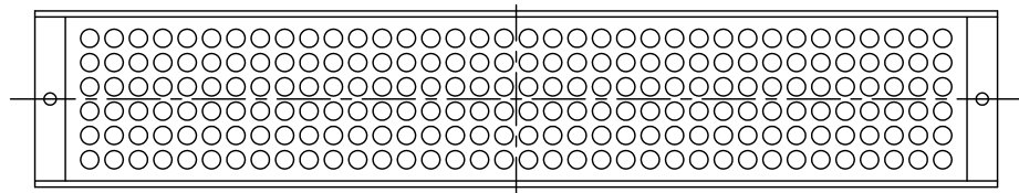
赤, 赤外 照明 36個x6列 (素子間P=4mm)
