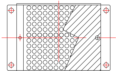
赤, 赤外 照明 12個x12列(素子間P=4mm)
