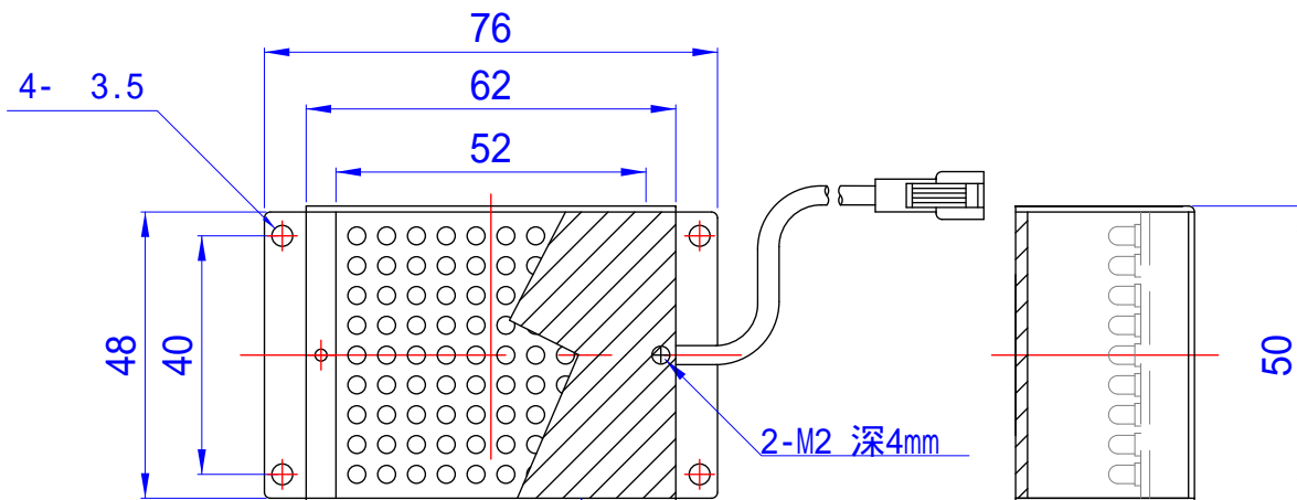
白, 青, 緑, 紫外 照明 10個x9列(素子間P=5mm)
