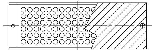
赤, 赤外 照明 18個x6列 (素子間P=4mm)
